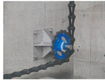
角軸鏈輪 (污泥坑處)
