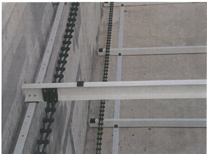
上方回程導板, 下方磨耗軌道
